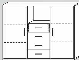
60313/40/F/G* 134x102x40cm (BxHxT) 60313/32/F/G* 134x102x32cm (BxHxT)
