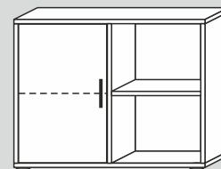
60108L/40/F/G* 90x70x40cm (BxHxT) 60108L/32/F/G* 90x70x32cm (BxHxT)
