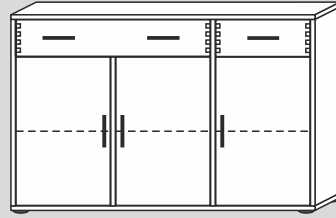
60300L/40/F/G* 134x86x40cm (BxHxT) 60300L/32/F/G* 134x86x32cm (BxHxT)
