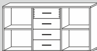
60264/40/F/G* 134x70x40cm (BxHxT) 60264/32/F/G* 134x70x32cm (BxHxT)
